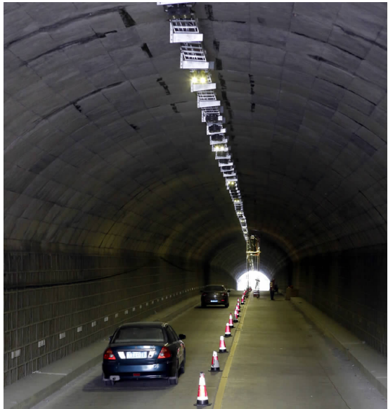
11月18日,千威线上的一个隧道内在安装LED照明灯
